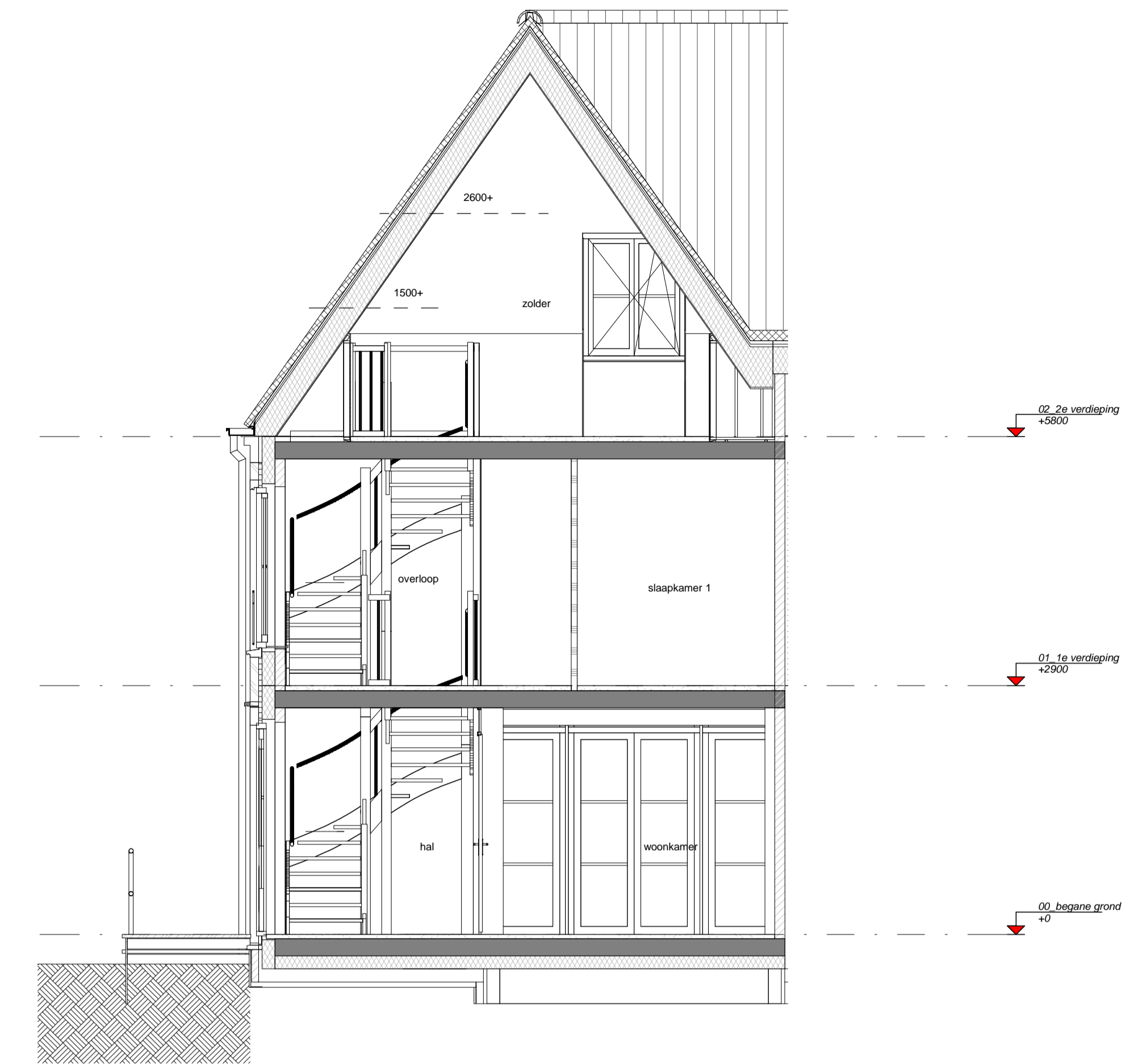
doorsnede B-B schaal 1 : 50
