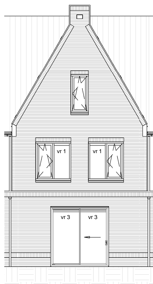
Achtergevel
