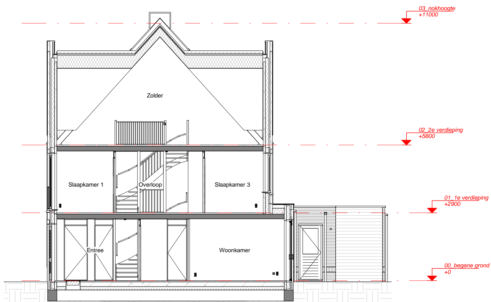
Doorsnede
