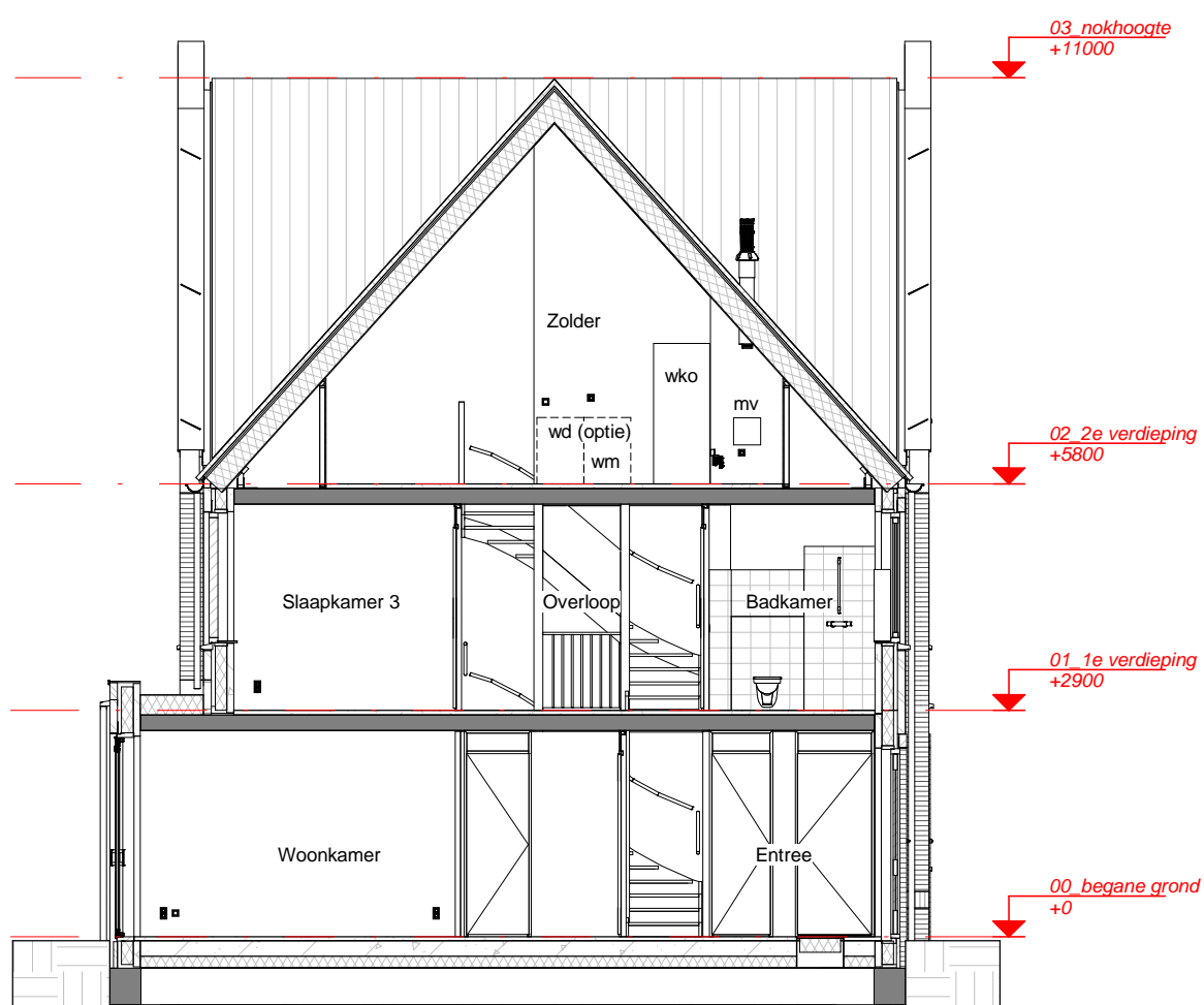
Doorsnede
